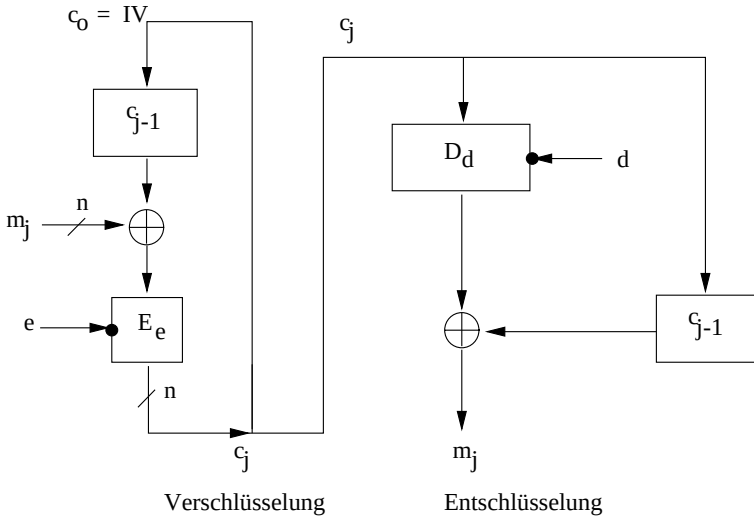
Abb. 4.2. CBC-Mode
